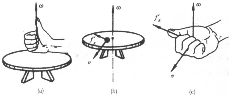
图 1.5 角速度和科里奥利力方向的判断
