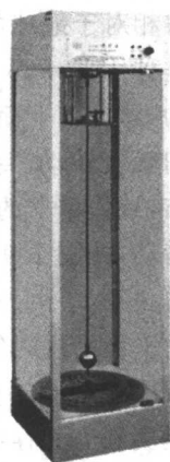
图 1.6 傅科摆
