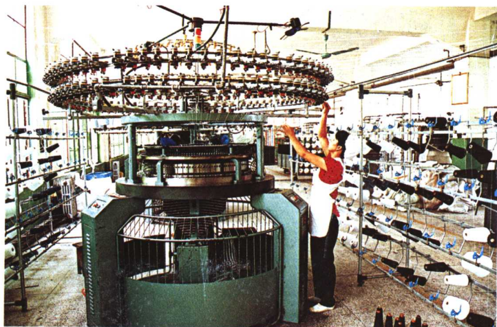
◀南平针织厂针织大圆机
