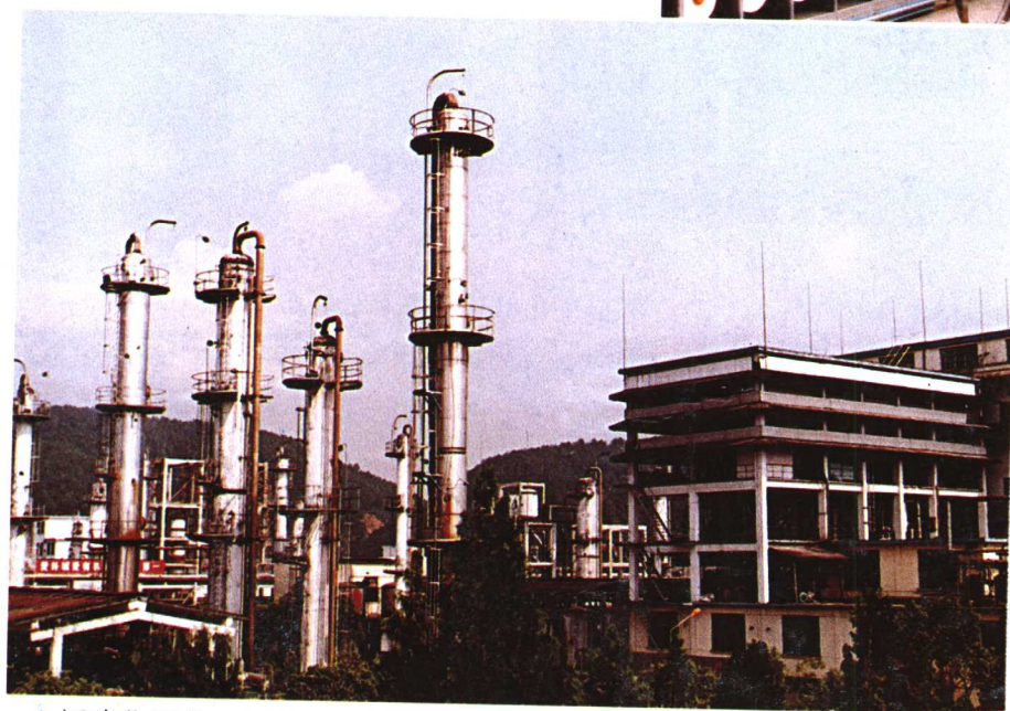
▲ 福建化纤化工厂聚乙烯醇车间
