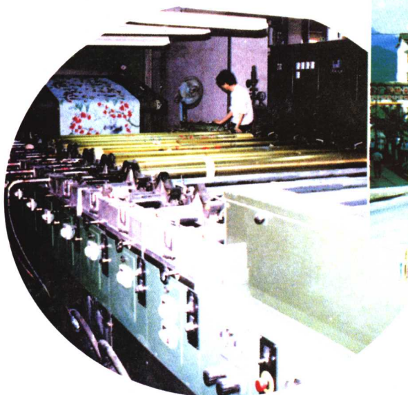
▲三明印染厂 12 套色圆网印花机
