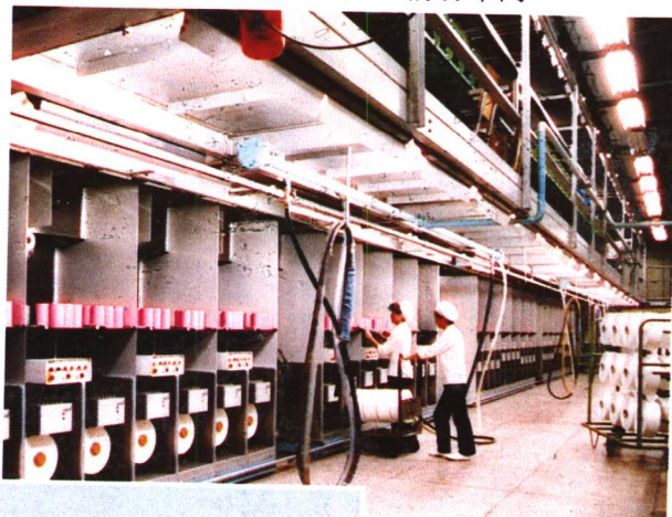
▼ 福建化纤化工厂涤纶分厂前纺车间
