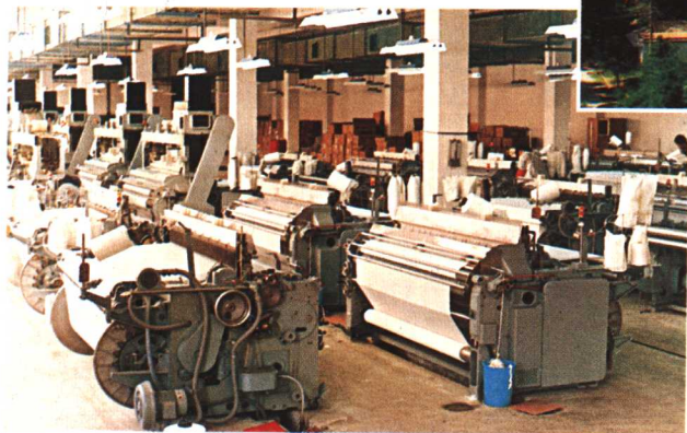
▼ 厦门纺织厂喷水织机车间
