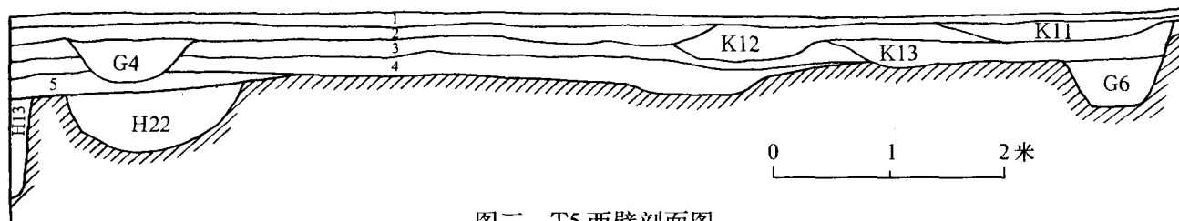
图三 T5西壁剖面图
