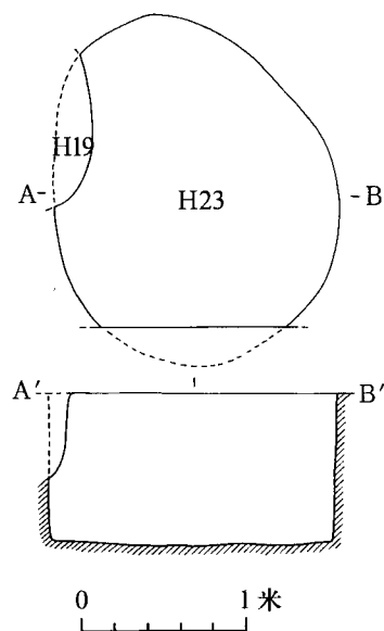
图六 H23平、剖面图
