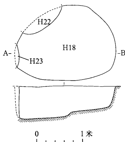
图七 H18平、剖面图
