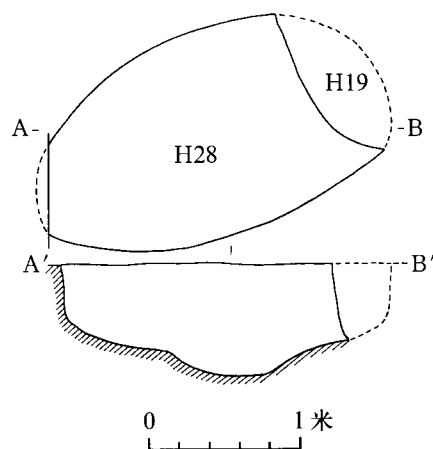
图八 H28平、剖面图
