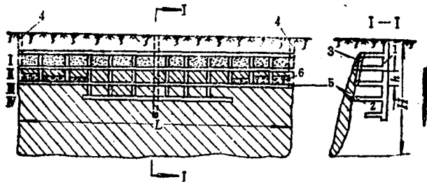
图 2-2 阶段和矿块的划分
