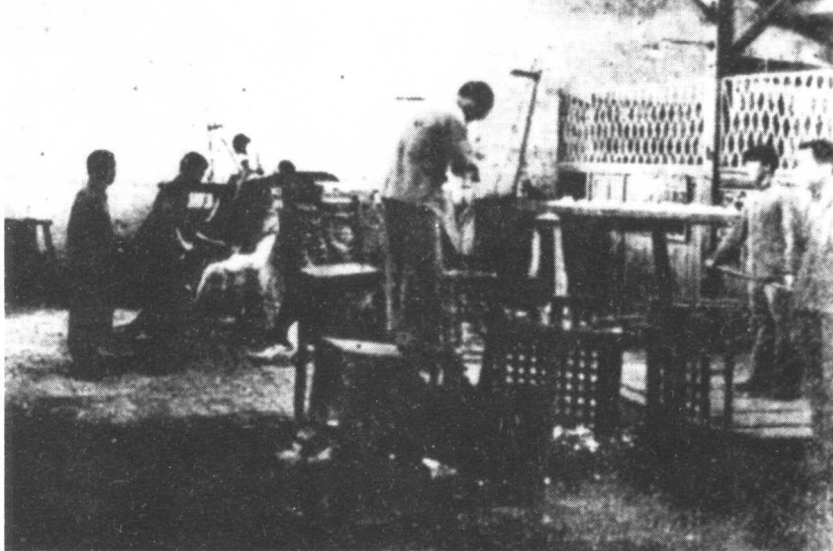
亚浦耳工人 吹制灯泡时的工作情形。
