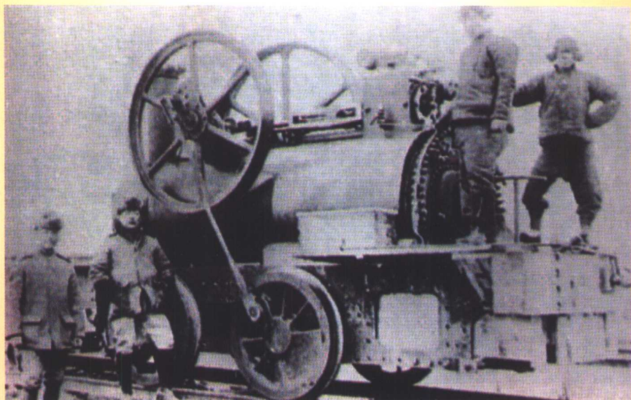
1881 年唐胥铁路通车,图为中国人自己制造的第一台蒸气机车
