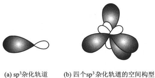
图 1-1 碳原子的 sp^3 杂化
