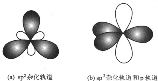
图 1-2 碳原子的 sp^2 杂化
