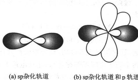
图 1-3 碳原子的 sp 杂化
