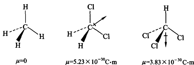
图 1-4 几种化合物的偶极方向和偶极矩
