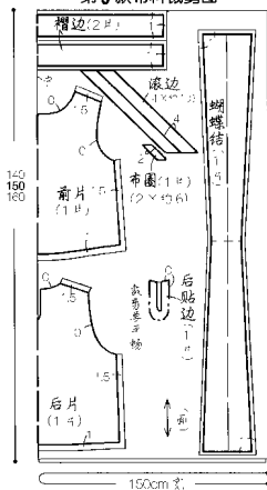
第3款布料裁剪图
