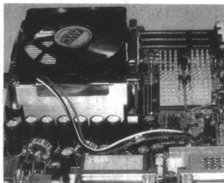
图 1.2 安装 CPU 散热器
