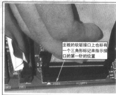
图 1.21 把软驱数据线插入 FDD 插槽中
