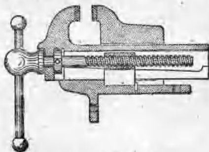
圖 4. 虎鉗構造圖
