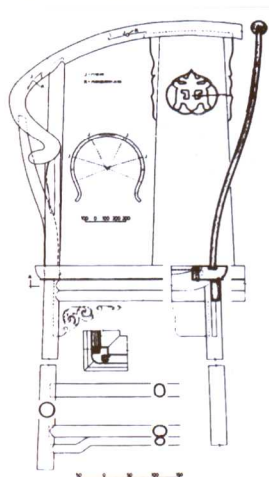
明 圈椅结构图
