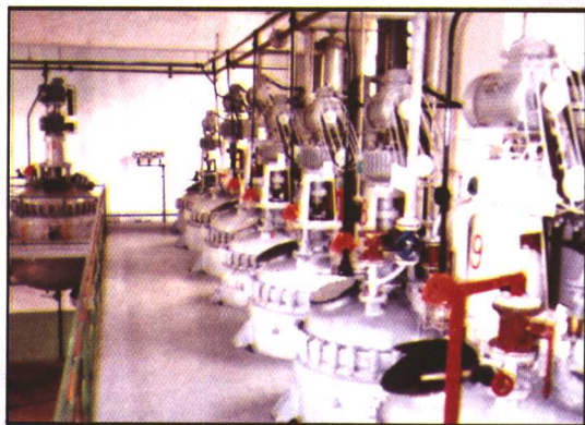
烟酰胺生产线(厦门第二制药厂) ▶
