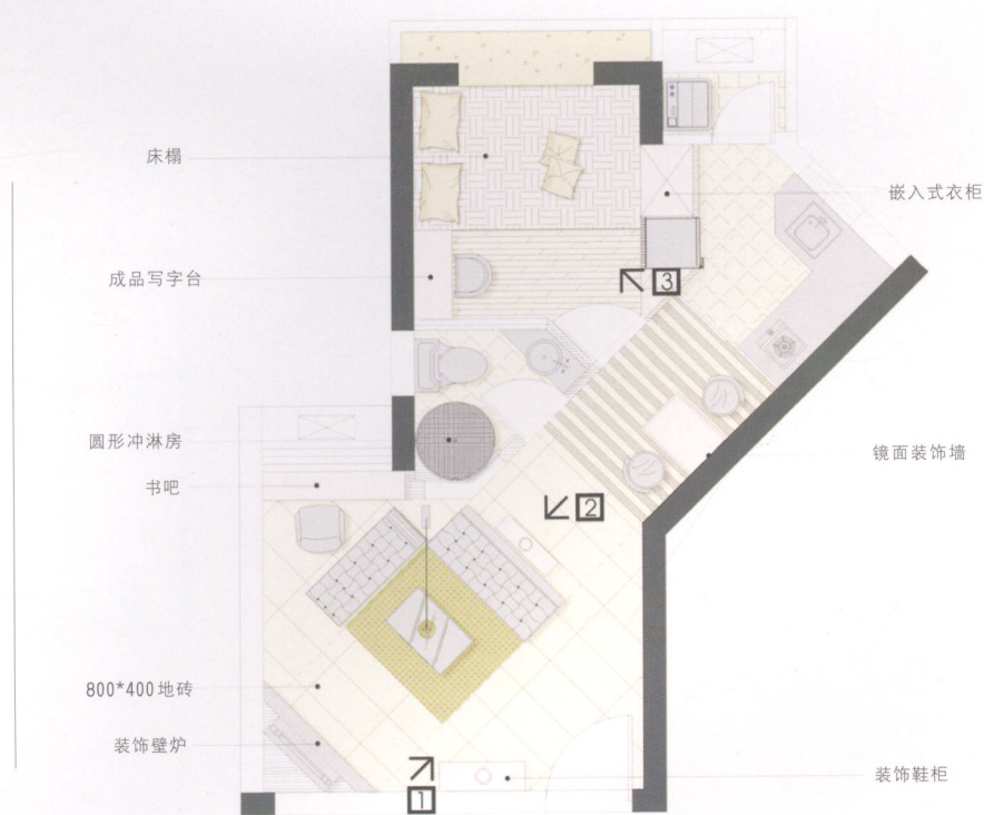
▲ 平面图
