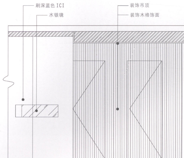
▲ 走道立面图
