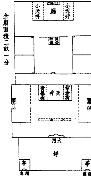
宗廟平面圖
