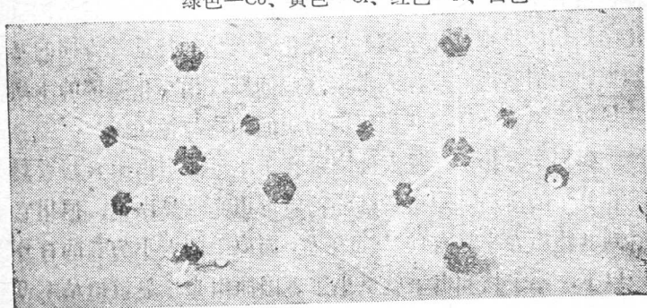
顺式
