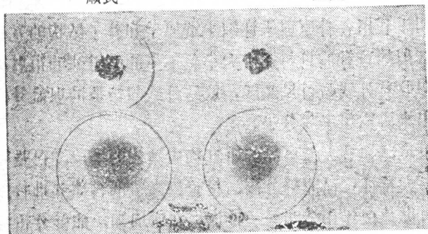
顺式
