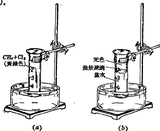
图 1·2 甲烷和卤素的取代反应实验
