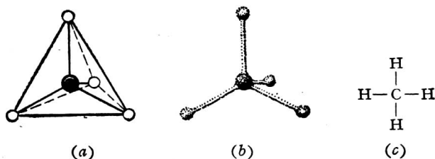
图 1·1 甲烷的分子结构
