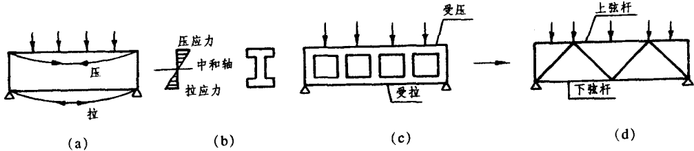
图 1.7 由简支梁发展成为桁架
