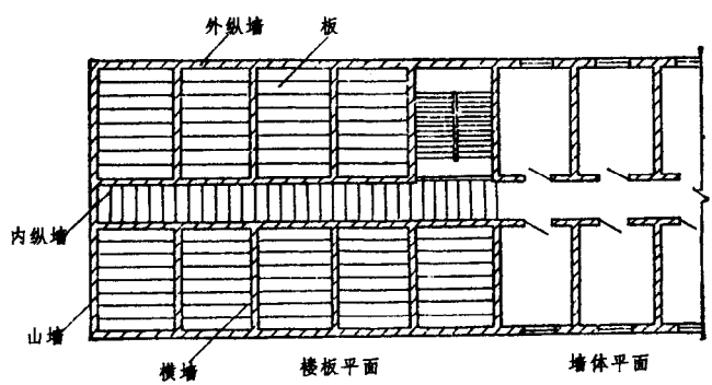
图 1.8 横墙承重方案
