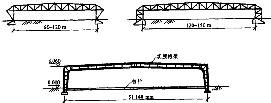
图 1.15 格构式刚架结构及实腹式双铰刚架
