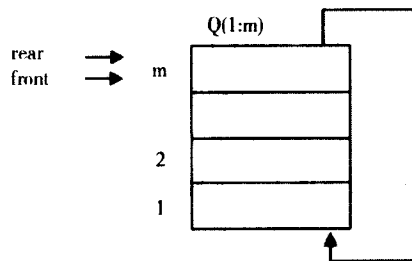
图 1-11 循环队列存储空间示意图
