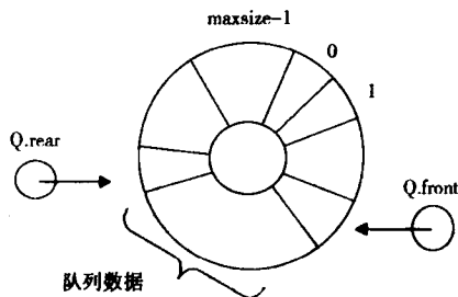
图 1-12 循环队列示意图
