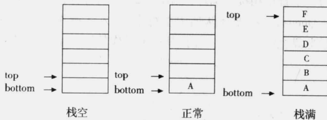
图 1-8 栈的状态
