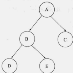
图 1-2 树型结构
