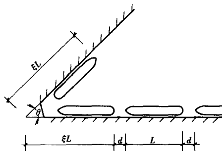
图 4.3.8-1 直立式岸壁折角处的泊位长度
