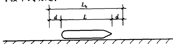
图 4.3.6 单个泊位长度
