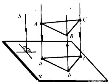
图 0-4 正投影法
