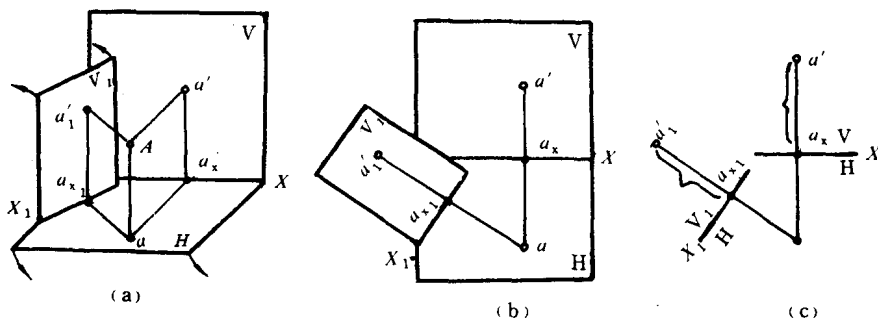
图 1-5 点对辅助投影面 V_1 面的投影
