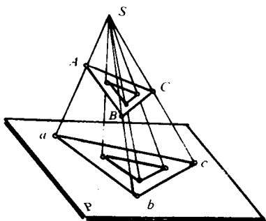
图 0-2 中心投影法
