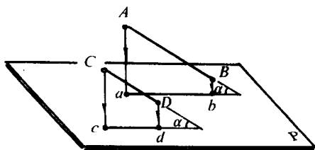
图 0-6 平行线段的投影
