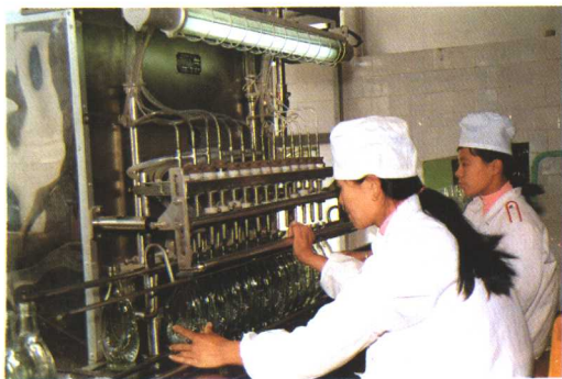
莱州特曲包装流水线
