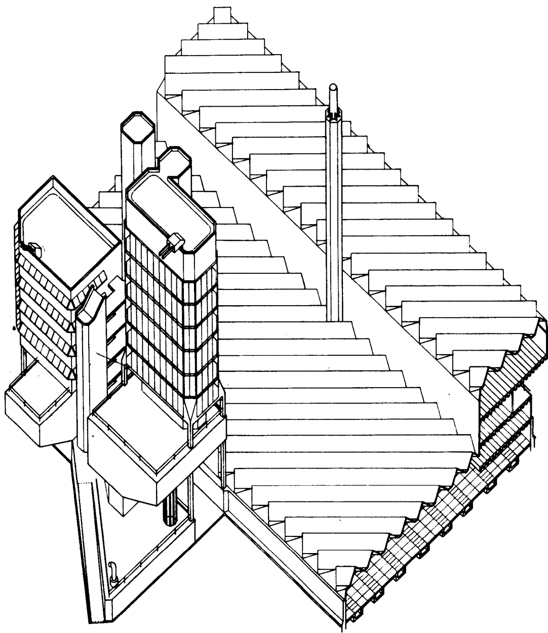
轴测表现图 詹姆斯·斯特林、詹姆斯·高恩 (James Stirling, James Gowan), 1959
