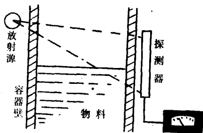
图1.1 \gamma 射线物位计测量原理
