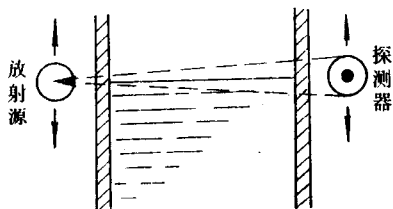
图1.5 随动式 \gamma 射线物位计
