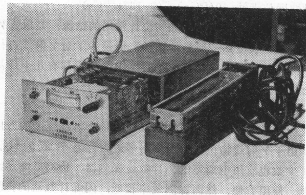
图1.2 \gamma 料位控制器
