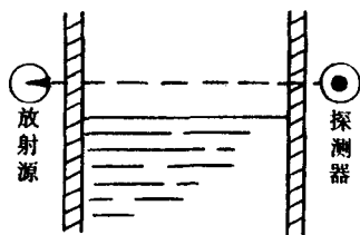
图1.3 \gamma 继电器工作原理图
