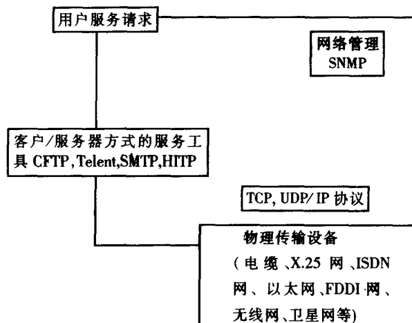
图 1-2 Internet 结构
