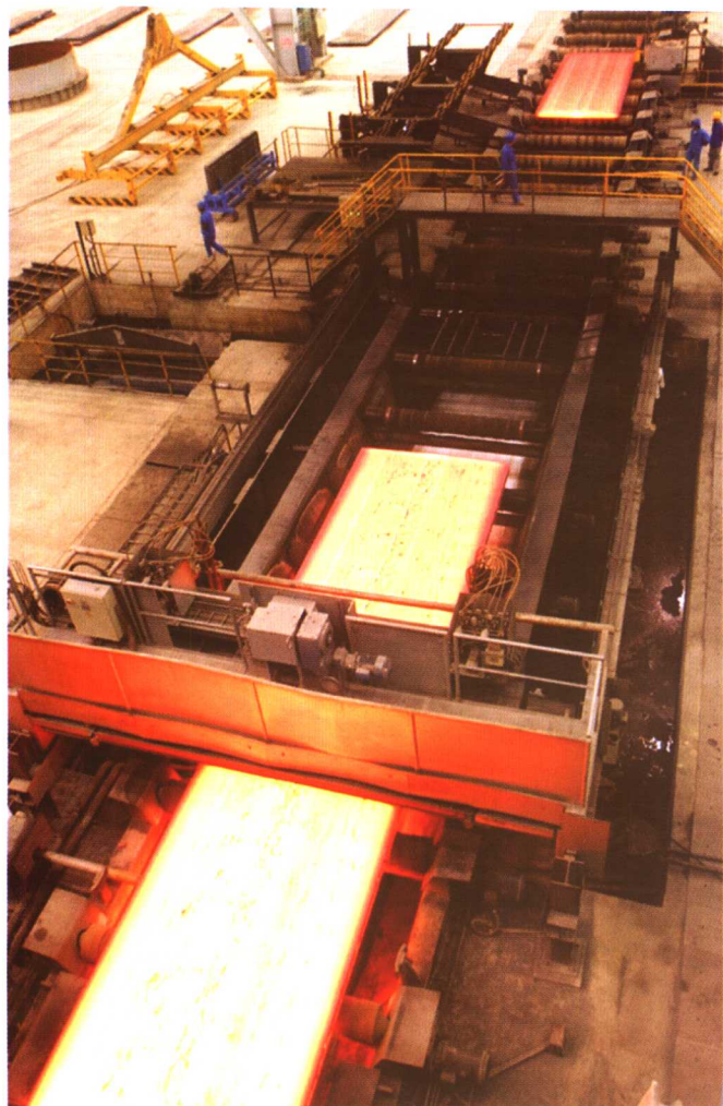
2004年10月，具有国际一流水平的世界第一条转炉——炉卷轧机生产线在南京钢铁有限公司建成后正式投产。图为新建成投产的3250宽厚板坯连铸机生产线。
