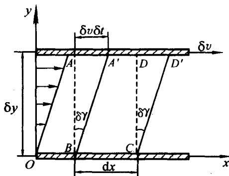
图 1.5 黏性
