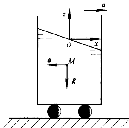
图 1.2 重力和惯性力
