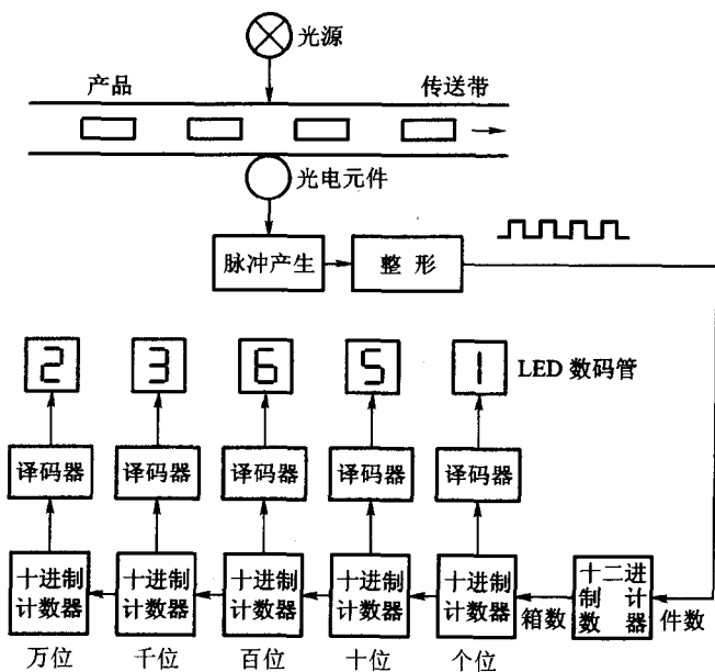
图 0.3 产品自动装箱计数生产线
