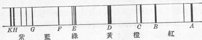
圖 25-5 太陽光譜的可見光部份中的 夫牢因 和 斐 暗線，這兒只畫了最顯然的線中的幾條。
