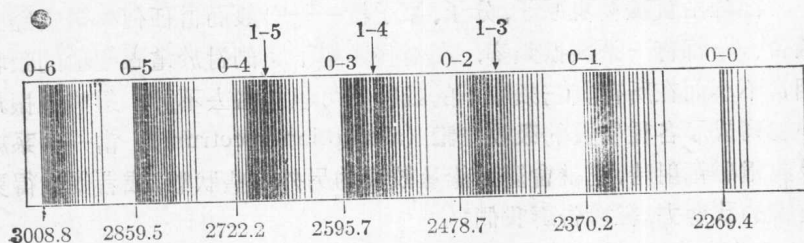
圖 25-3 簡化了的 一氧化氮(NO) 的分子光譜，自 3100 埃到 2100 埃。下面的數目是每一個帶頭上的波長，上面的數目是產生遷徙的振動階的被指定值。〔自由地從 Spectra of Diatomic molecules, G. Herzberg New York D. van Norstranel Co. 1950. 這書中採用的〕。
