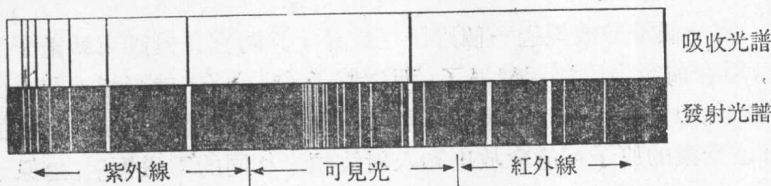
圖 25-4 鈉蒸汽的吸收光譜線和放射光譜線的比較。〔借自 A.B. Avons, Development of Concepts of Physics, Addison-Wesley, 1965〕。
