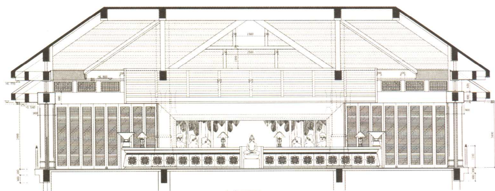
大堂立面 1
