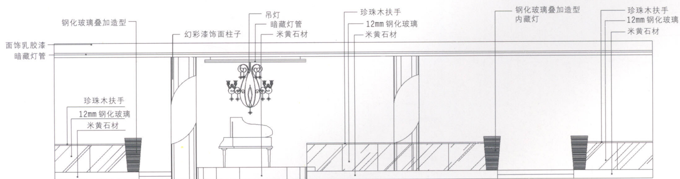
▲ 西餐厅立面图 B
