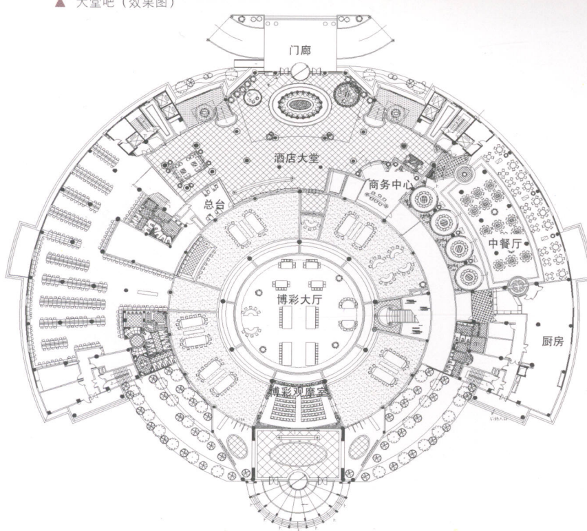
▲ 一层平面图
