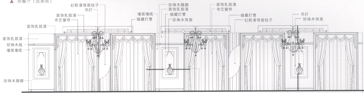
▲ 西餐厅立面图 A
