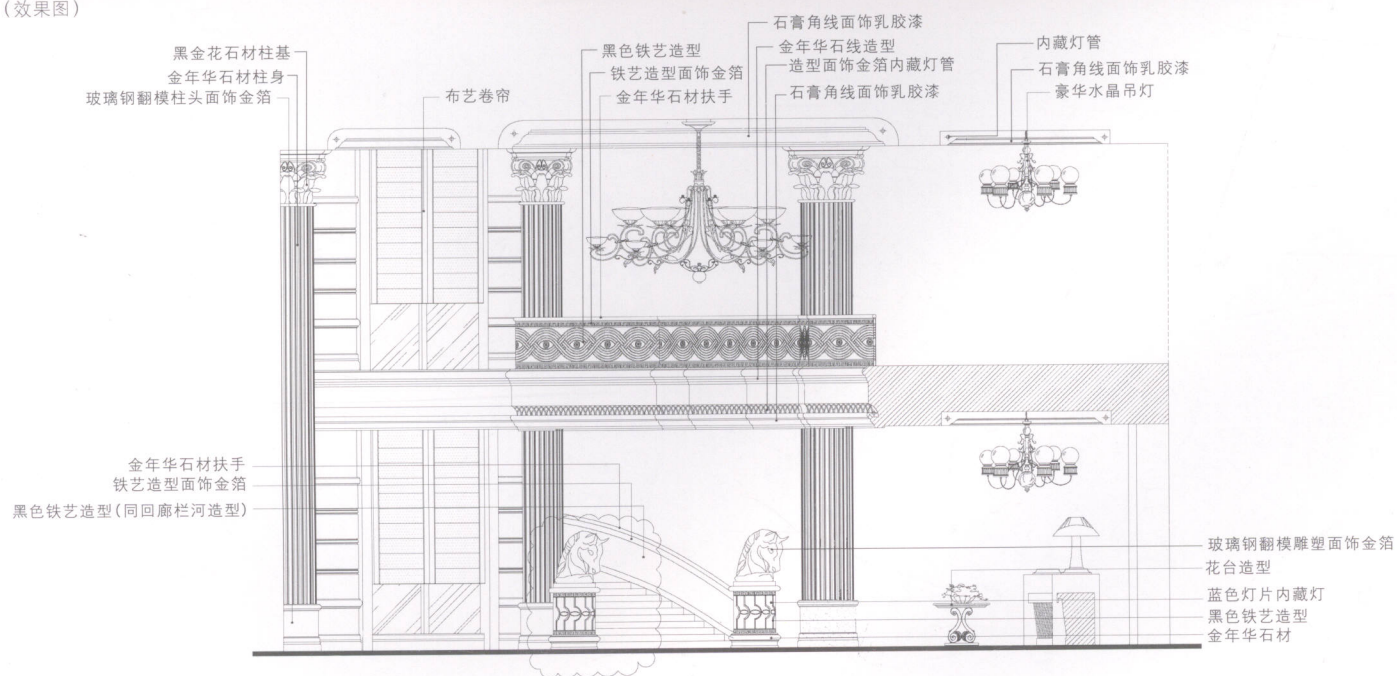
▲ 大堂立面图B
