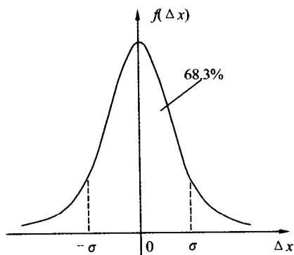
图 0-1 随机误差的正态分布
