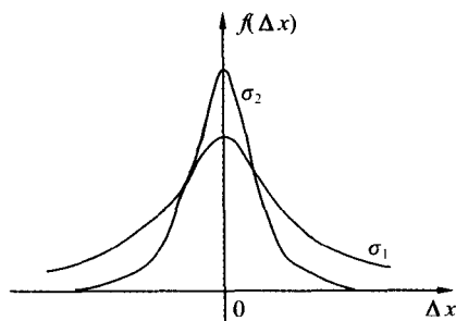
图 0-2 不同 \sigma 的概率密度曲线
