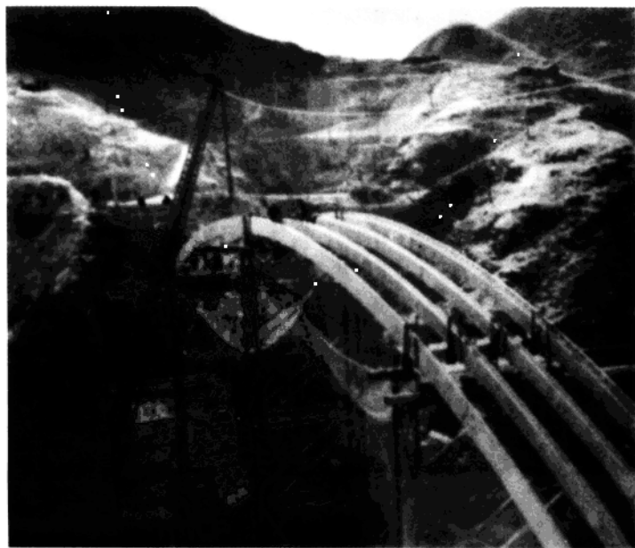
红旗渡槽正在施工中
