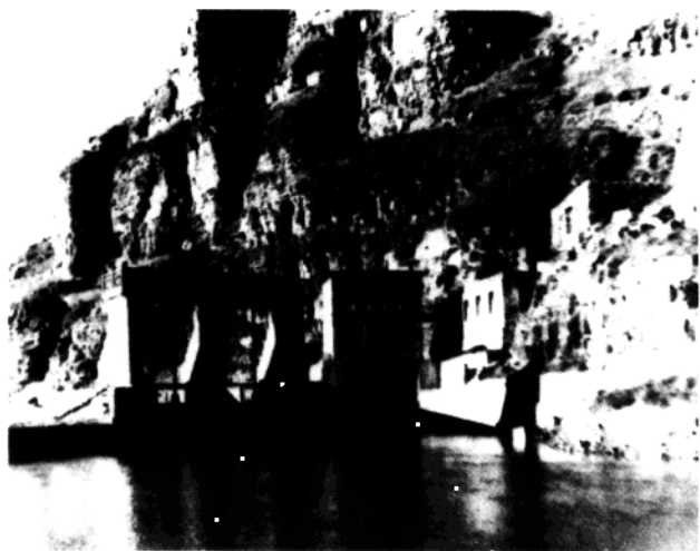
跃进渠首进水闸和泄洪闸
