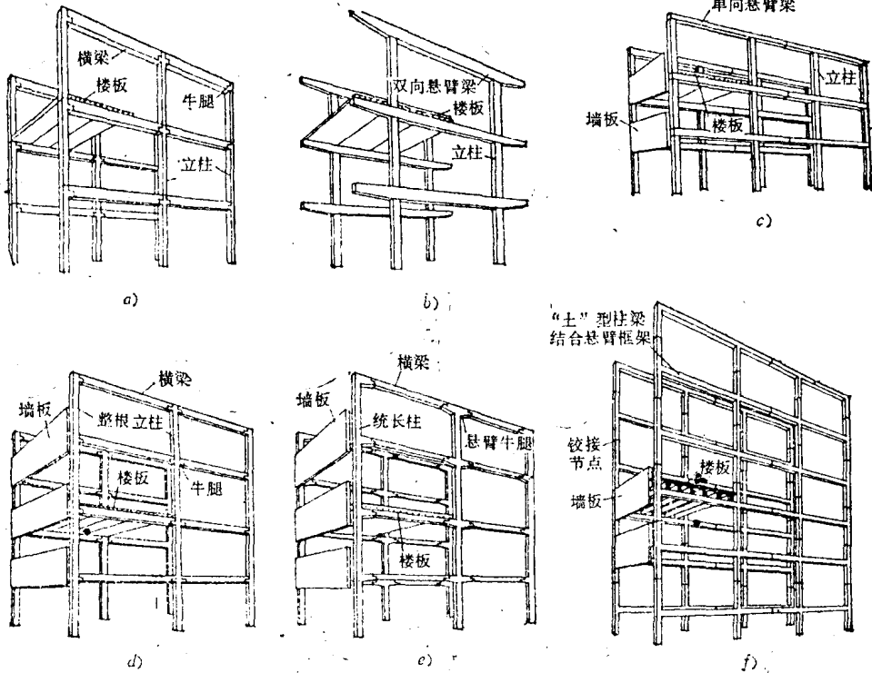
图 1-5 装配式横向框架的形式
