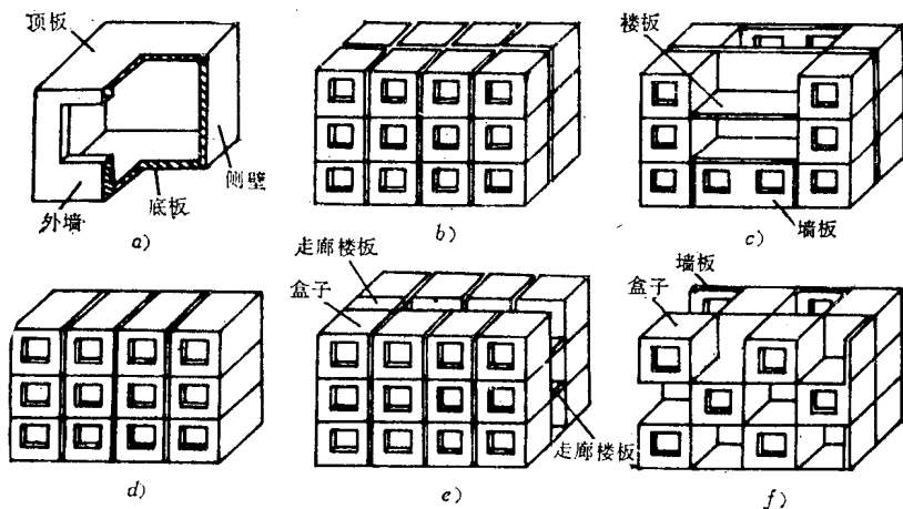
图 1-7 盒子结构建筑类型
