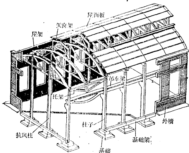
图 1-2 单层钢筋混凝土厂房的组成
