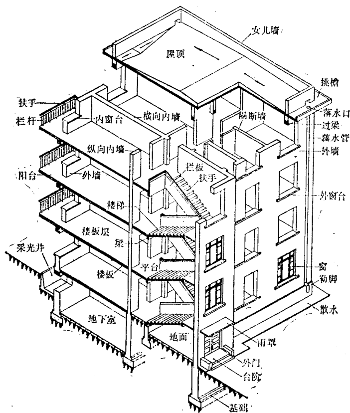
图 1-1 民用建筑的组成
