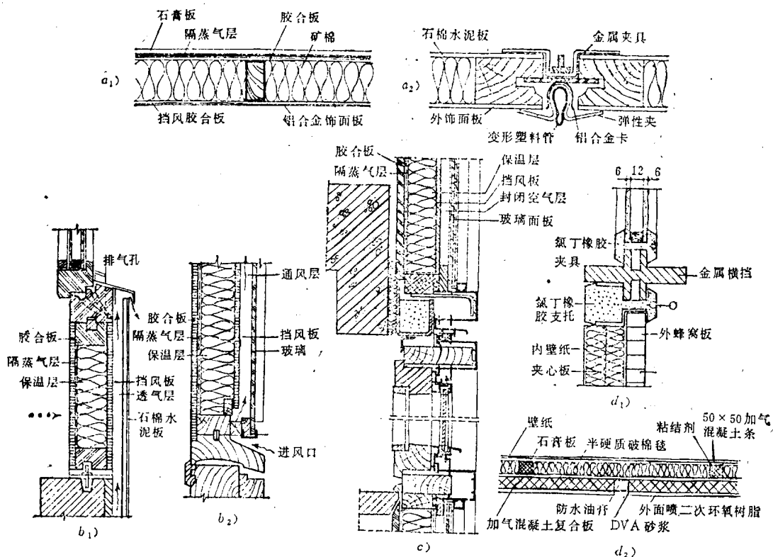
图 1-6 轻质外墙板组成和构造举例
