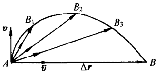
图 1-3 速度
