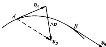
图 1-4 加速度
