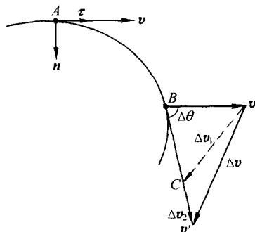
图 1-5 切向加速度与法向加速度
