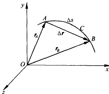
图 1-2 位移
