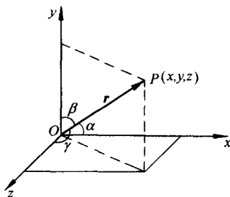
图 1-1 位置矢量
