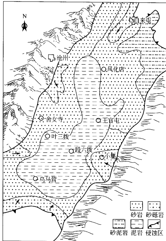
图 1-2 黄骠裂谷盆地孔店组二段沉积环境略图
