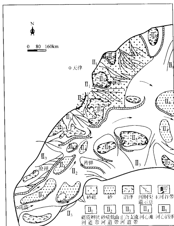
图 1-7 黄骅裂谷盆地馆陶组沉积环境略图
