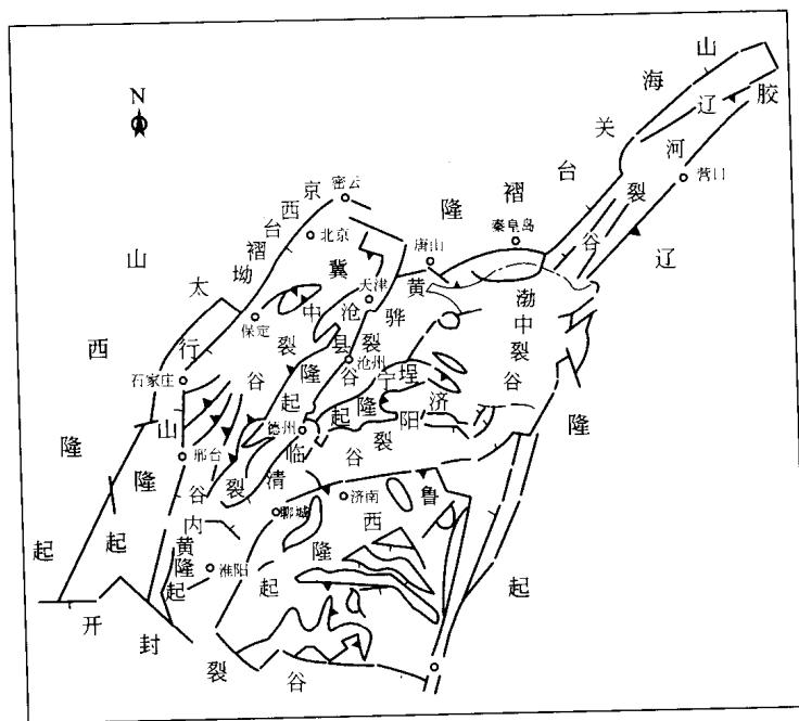
图 1-1 渤海湾裂谷盆地构造区划示意图
