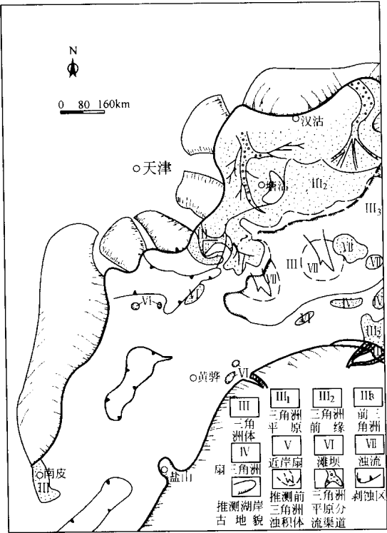
图 1-6 黄骅裂谷盆地东营组下段沉积环境略图
