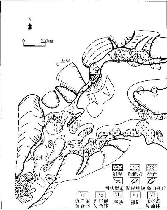
图 1-4 黄骅裂谷盆地沙河街组三段沉积环境略图
