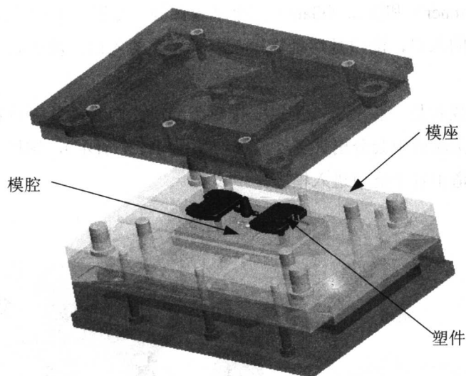
图 1.1.6 模座
