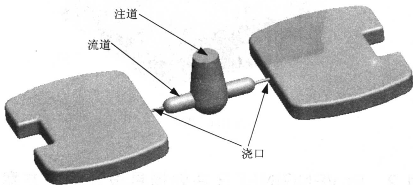
图 1.1.4 浇注系统
