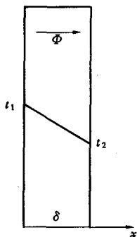
图1-1 大平壁的稳态导热
