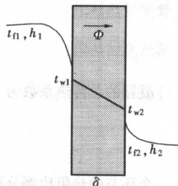
图 1-2 传热过程示意图
