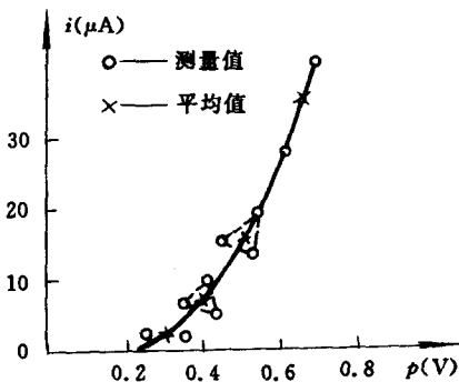
图 1.3.2 分组平均法修匀曲线
