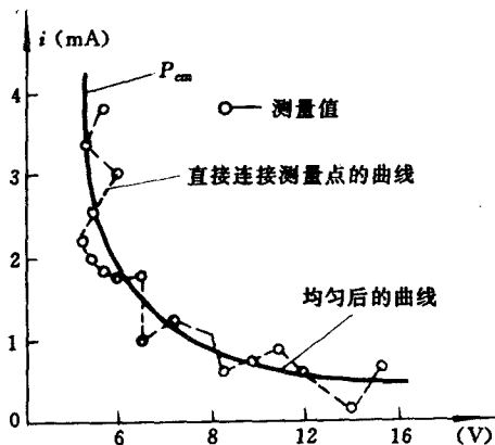
图 1.3.1 直线连接测量点时曲线的波动情况
