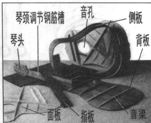
民谣吉他内部结构图
