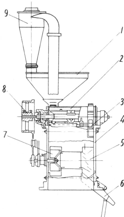
结构示意图
