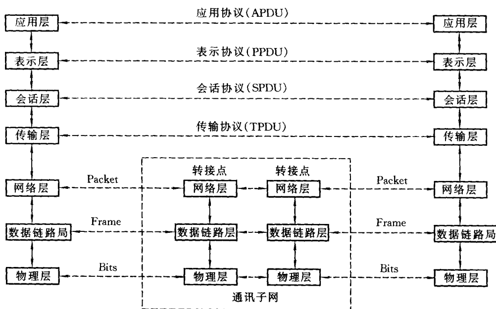
图 1.3 7 层 OSI 参考模型
