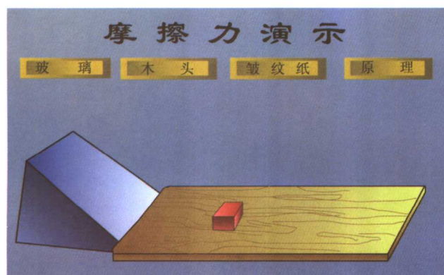
摩擦力演示
