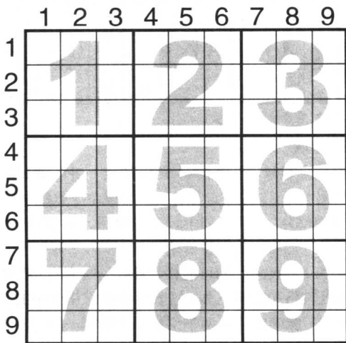
图1 示意九宫格坐标和小九宫格标号的空白数独
