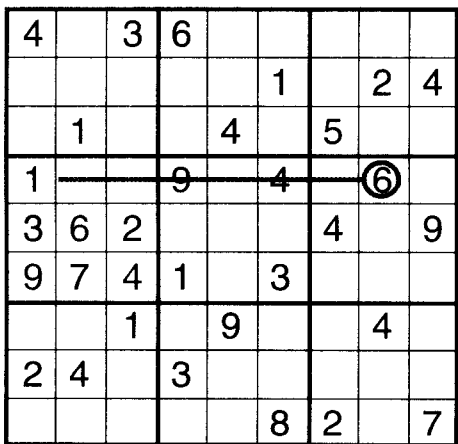
图6 方格(4, 8)的6表示小九宫格④中的6只可能出现在(5, 2)
