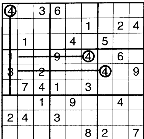
图5 找4以解答谜题
