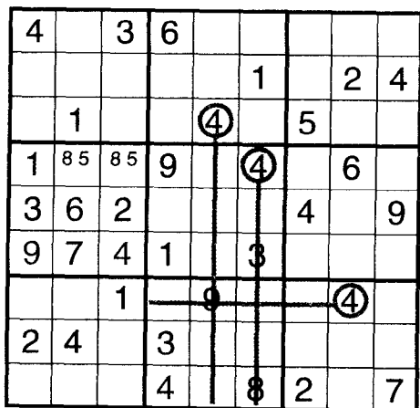
图7 分离出“好”线索
