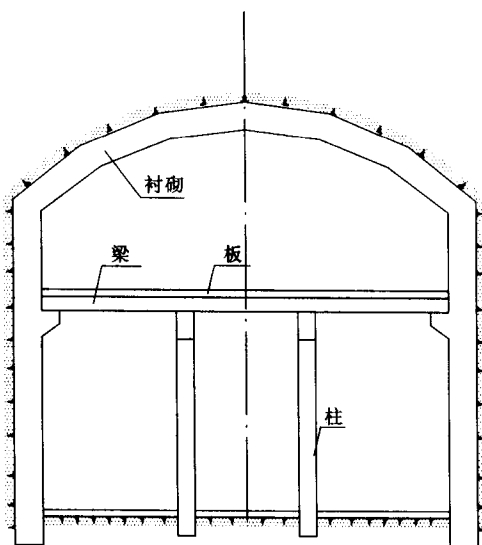
图 1-1 地下建筑图结构示意图
