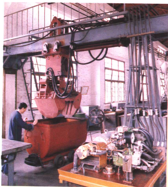
◁本省自行研制的全国 第一台液压矿用清车机
