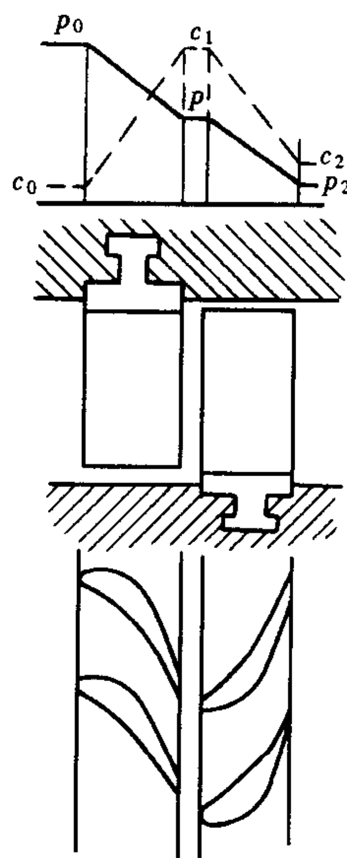
图 1-5 反动级中蒸汽压力速度变化示意图
