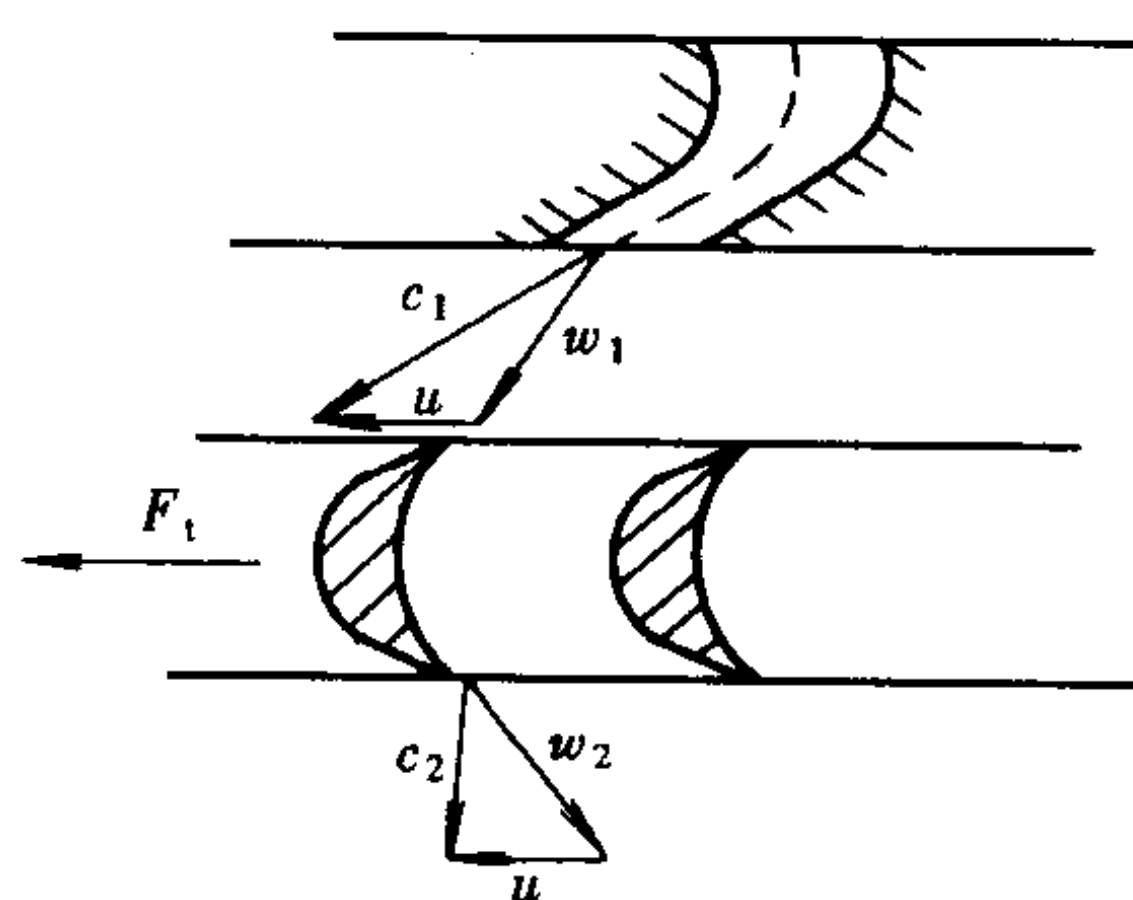
图 1-1 无膨胀动叶汽道内蒸汽的流动情况
