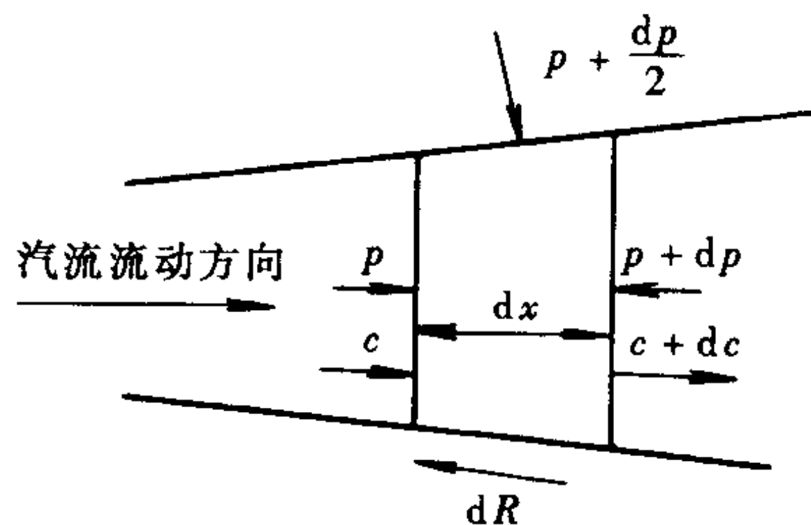
图 1-6 作用在汽流微元段上的力
