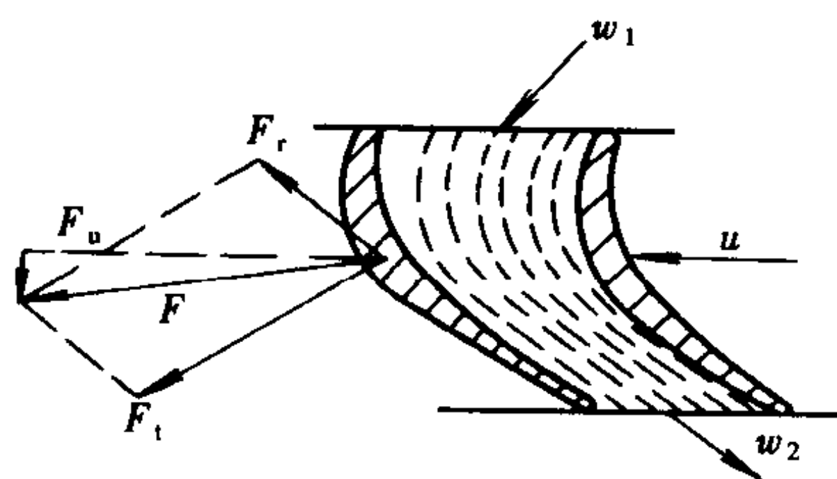
图 1-2 蒸汽在动叶汽道内膨胀的流动情况
