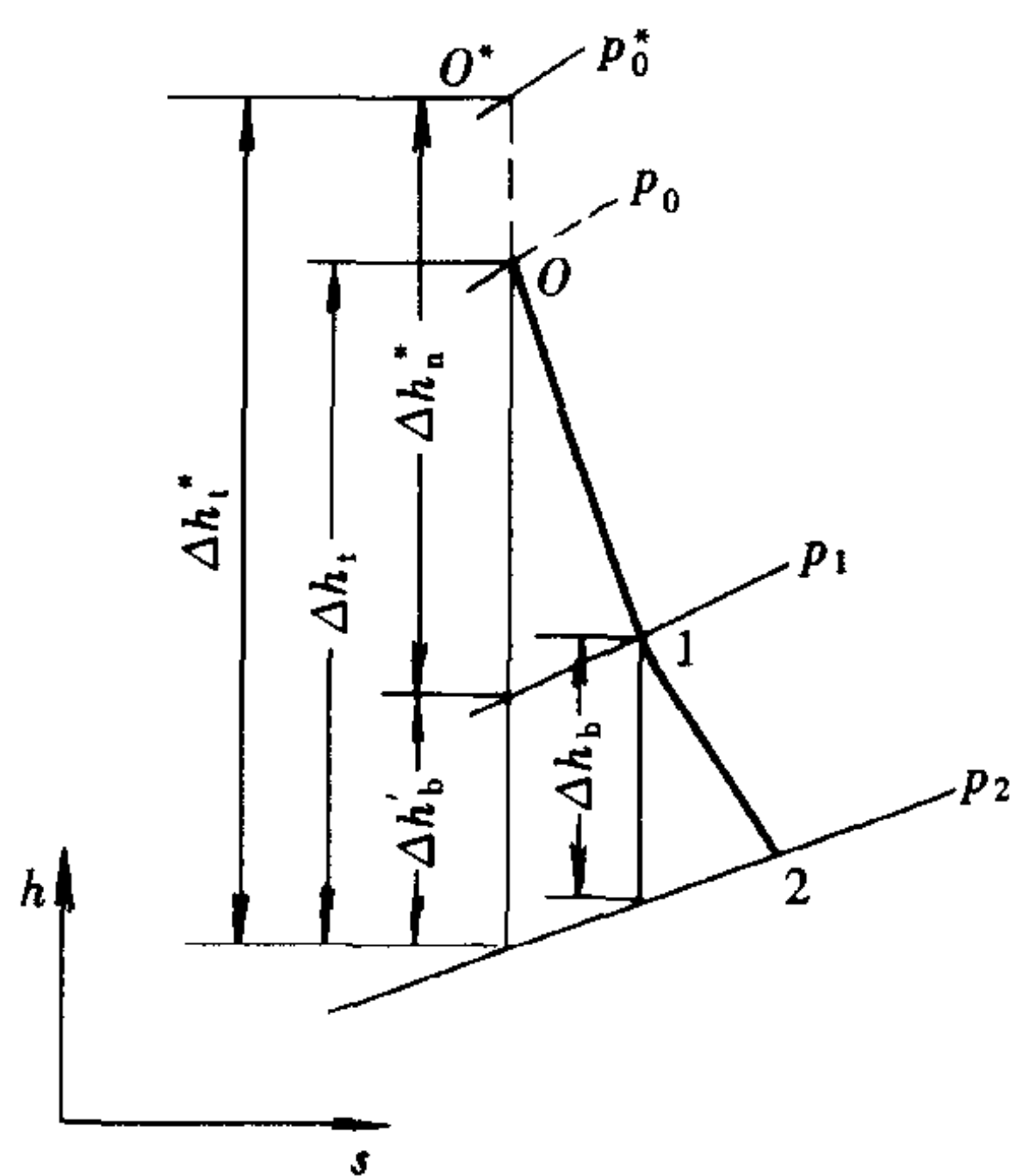
图 1-3 级的热力过程线
