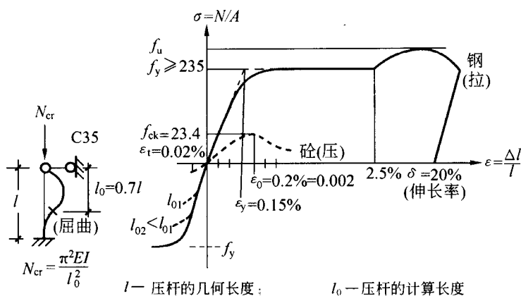
图 1-1 钢和砼 \sigma - \epsilon 曲线的比较
