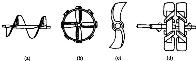
图 1-2 螺旋推进器初期的几种形式
