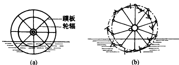
图 1-5 明轮推进器
