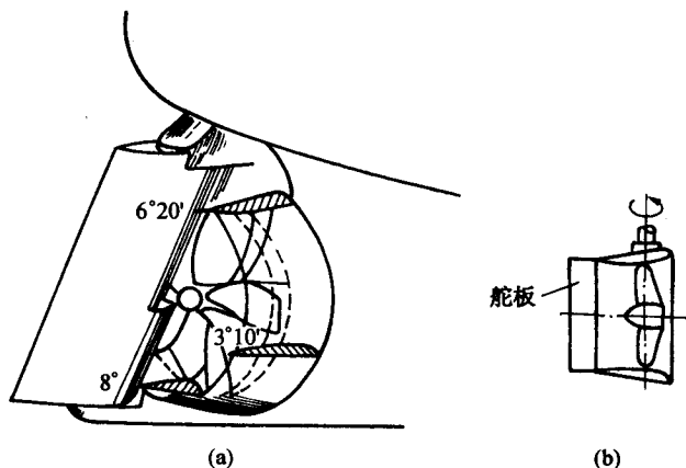
图 1-4 导管螺旋桨
