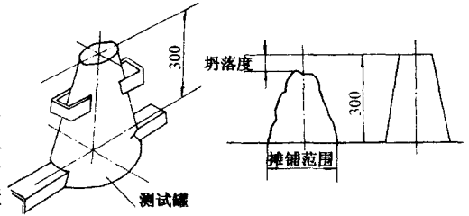
图 1-4 混凝土的坍落度和摊铺范围测试
