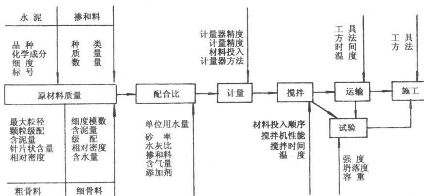
图 1-3 商品混凝土工厂生产工艺流程
