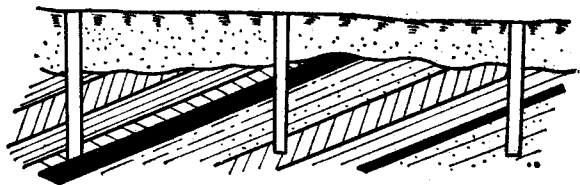
图 1—6 探井
