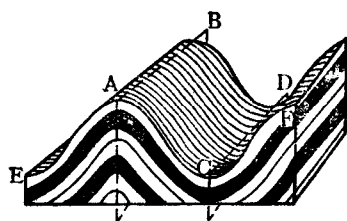
图 1—1 褶曲
