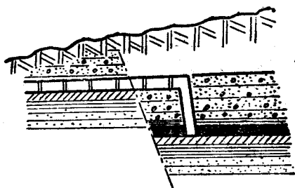
图 1—8 根据标志层及层位寻找煤层
