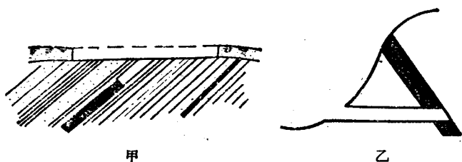
图 1—7 探峒
