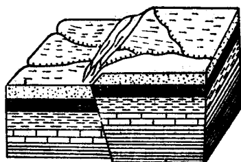
乙—逆断层
