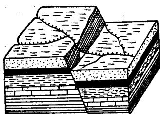
甲—正断层
