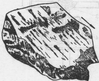
图1—12 擦痕
